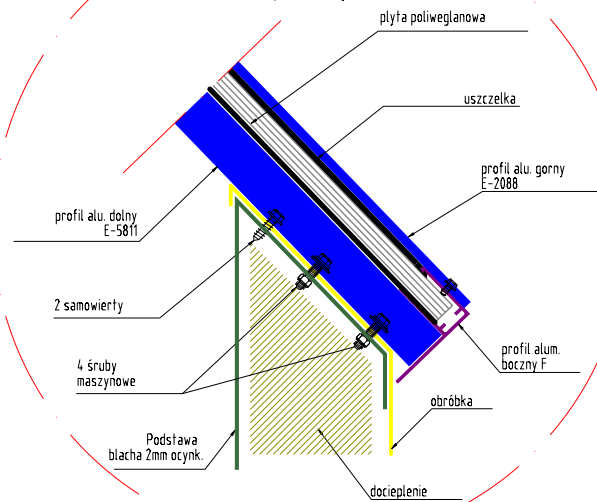
Mocowanie ścian bocznych świetlika do podstawy
