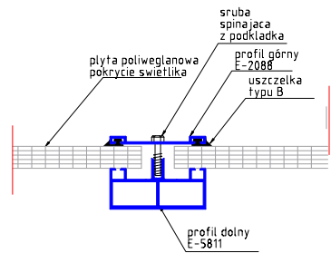
Połączenie płyt poliwęglanowych pokrycia świetlika
