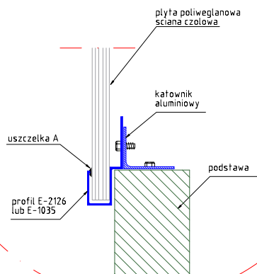
Mocowanie ściany czołowej świetlika do podstawy
