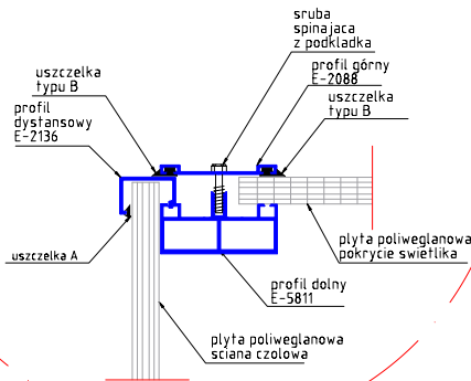
Mocowanie ściany czołowej z pokryciem świetlika
