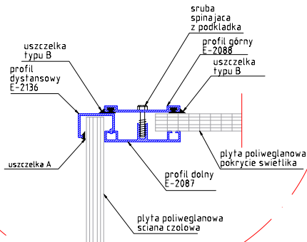
Mocowanie ściany czołowej z pokryciem świetlika
