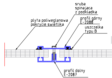
Połączenie płyt poliwęglanowych pokrycia świetlika
